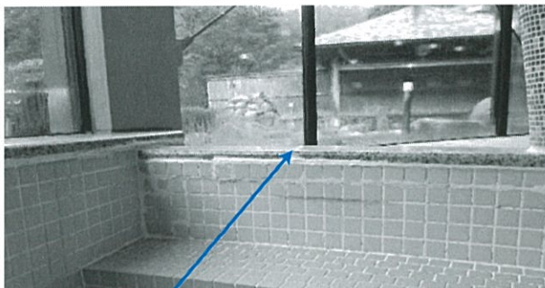
浴槽の歪みによるタイル変形
