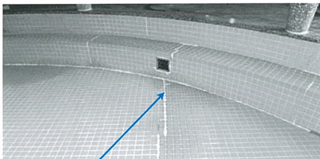
浴室床面の傾きによるヒビ発生
